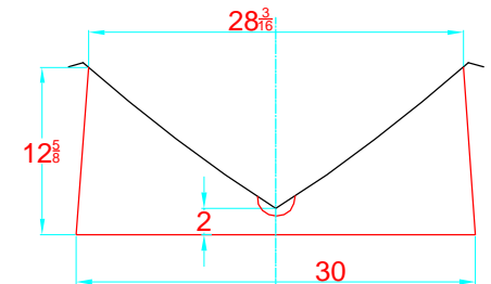
TRANSVERSAL SECTION "B" SECCION TRANSVERSAL "B"
